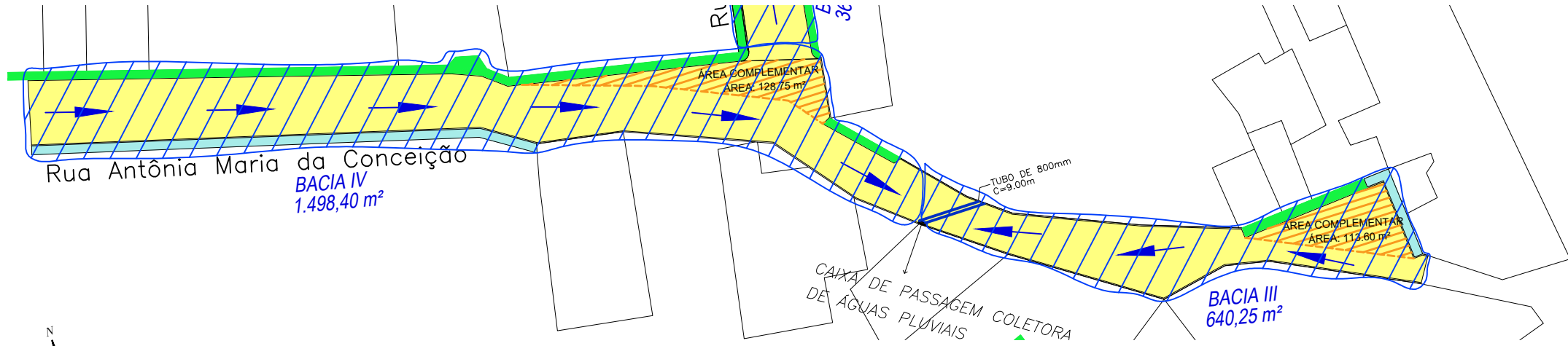
Drenagem Superficial das Águas Pluviais da Rua Antônio Maria da Conceição escala 1:750
