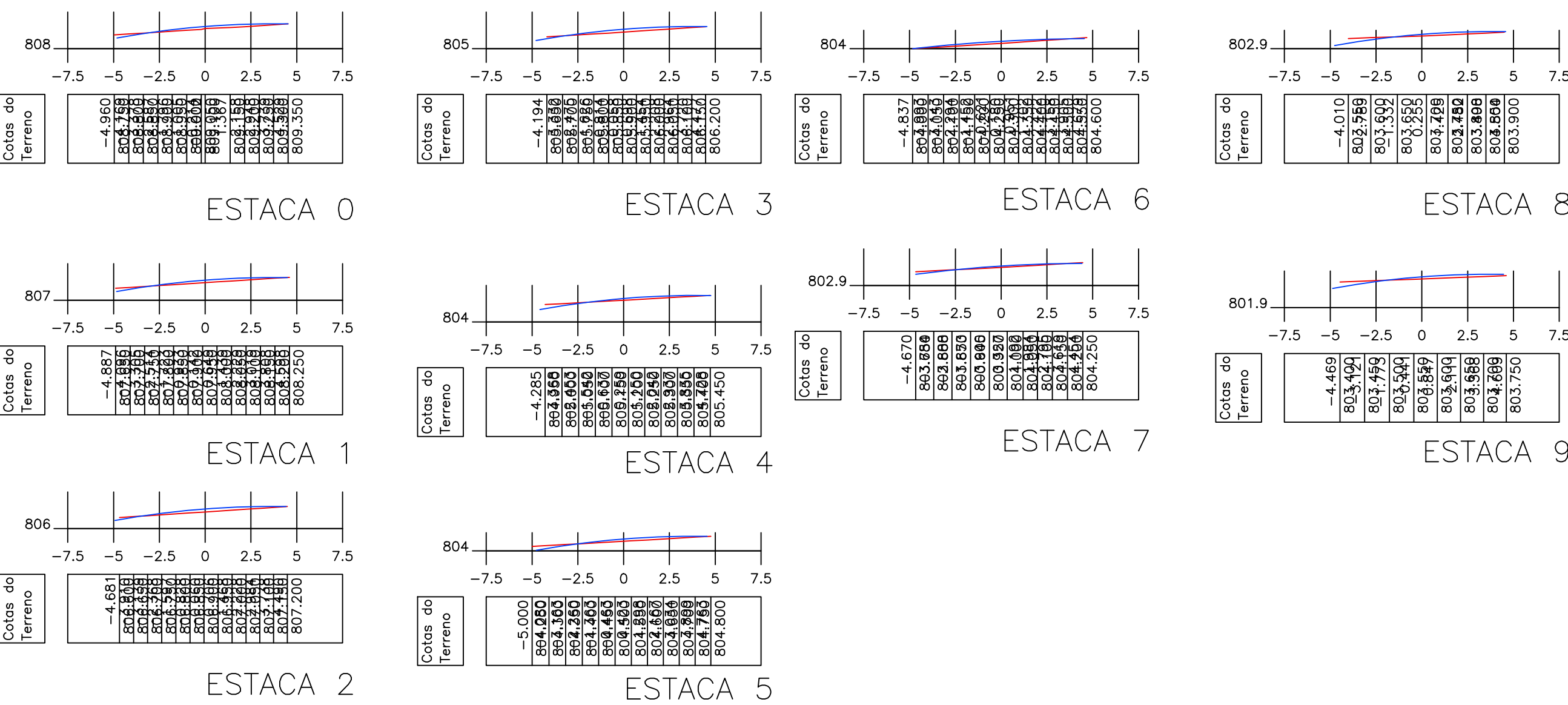
Seções Transversais da Rua Antônio Maria da Conceição
