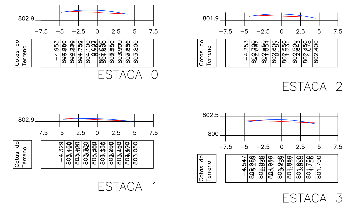
Seções Transversais da Rua João Vicente Gonçalves
