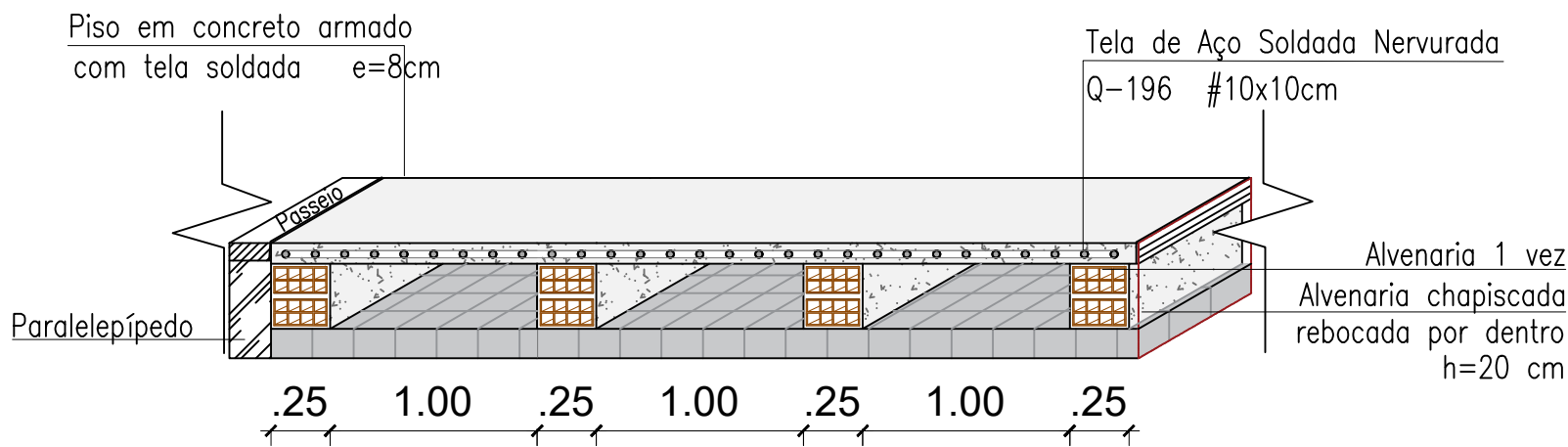
Perspectiva 01 - Entrada Lateral de Água escala 1:25
