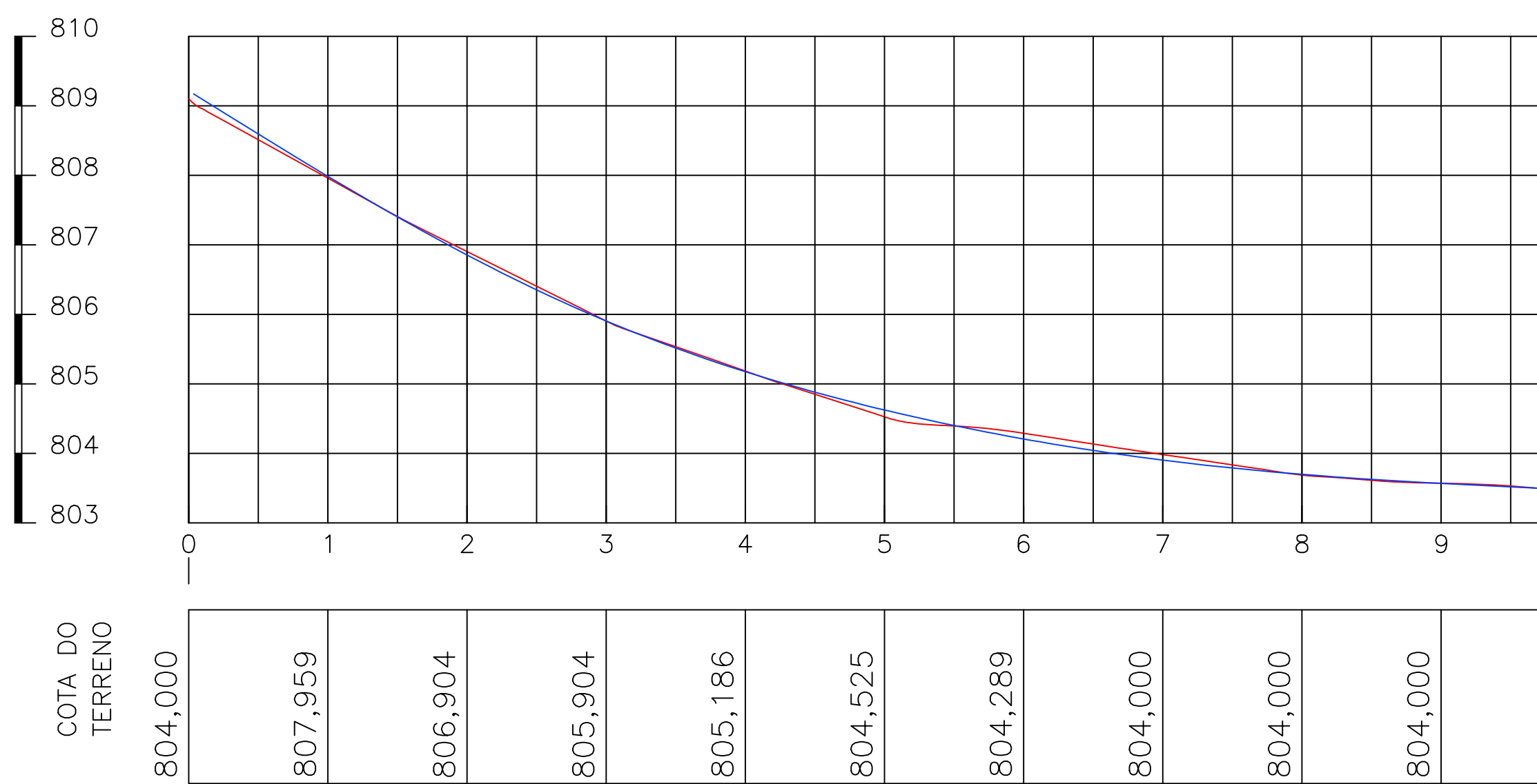
Perfil Longitudinal da Rua Antônio Maria da Conceição
