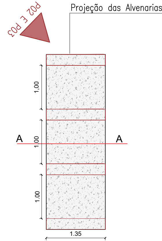
Vista Superior - Entrada Lateral de Água escala 1:50
