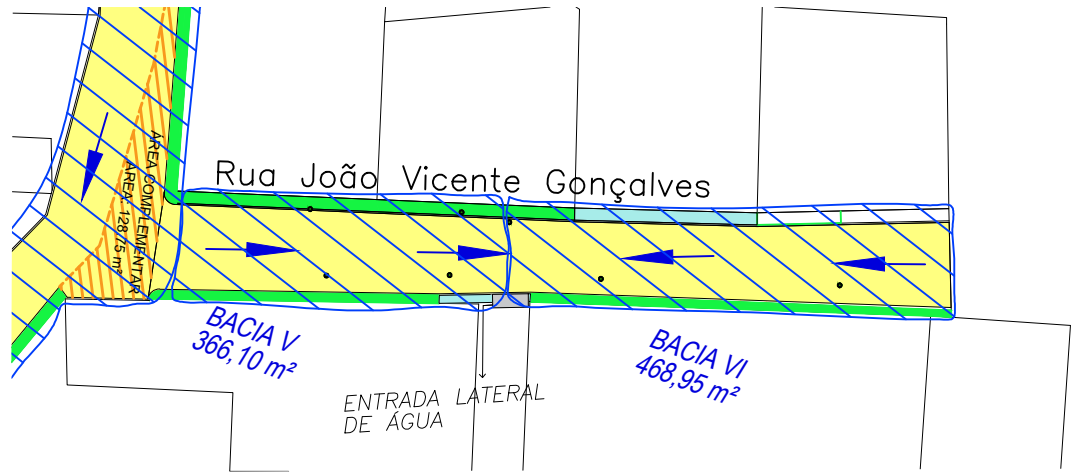
Drenagem Superficial das Águas Pluviais da Rua João Vicente Gonçalves escala 1:750
