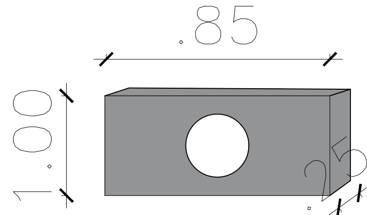
Detalhe da caixa de passagem coletora de águas pluviais escala 1:150
